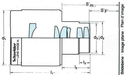
CINE-XENON 30-50 mm MC Ø 62,5
