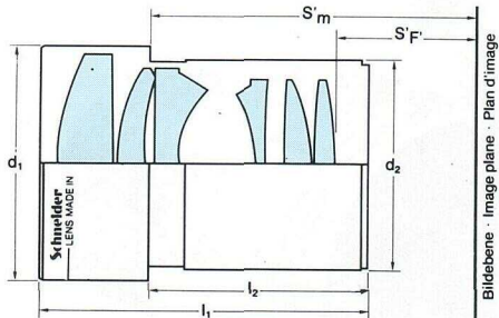
CINE-XENON 115- 150 mm MC Ø 62,5
