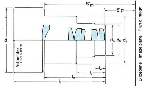
CINE-XENON 2/50 u. 55 mm MC Ø 70,65
